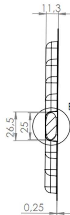
ŘEZ A-A
